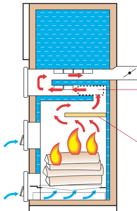
PUUOSAN POIKKILEIKKAUS
