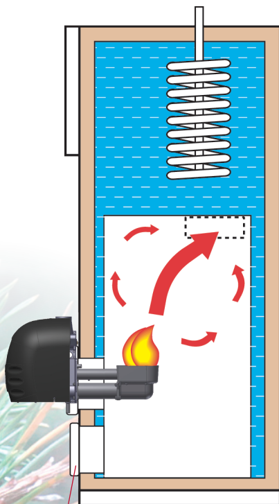
PELLETTIOSAN POIKKILEIKKAUS
